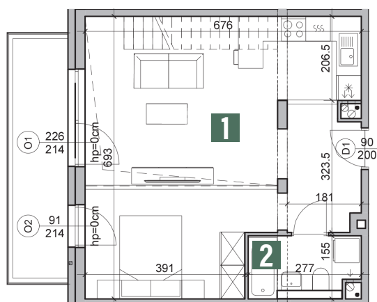
POZIOM 0 44,93m 2
