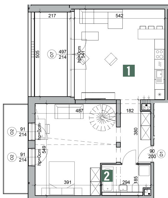
POZIOM 0 65,76 m 2
